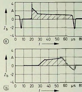
Bild 1. a) Basisstromverlauf des Transistors BU 108 bei 1,5 mA Strahlstrom, b) Basisstromverlauf in herkömmlichen H-Ablenkschaltungen
