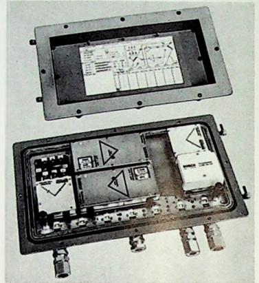
Kombinations-Verstärkergehäuse für das OGA-System (Bosch)
