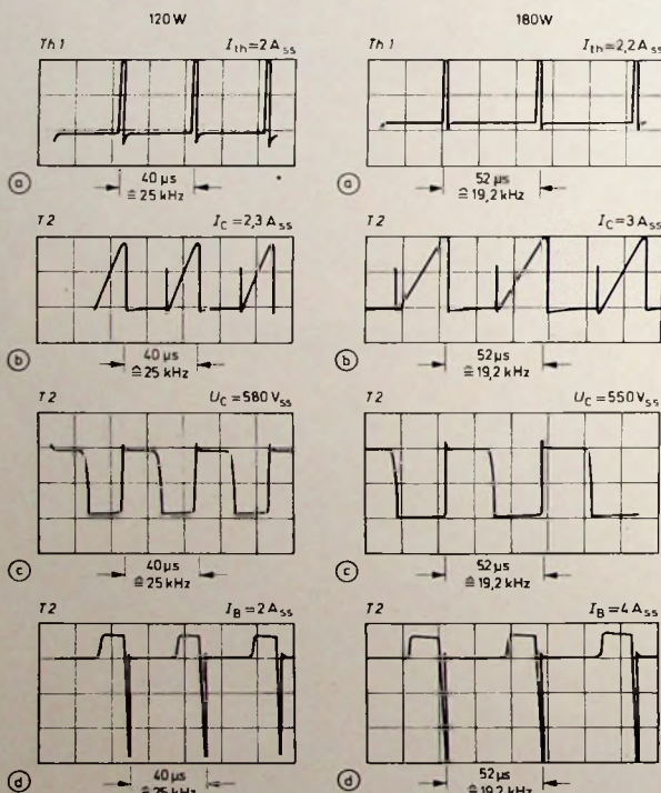
Bild 5. Freischwinger-Sperrwandlernetzteil für Volltransistor-Farbfernsehempfänger
