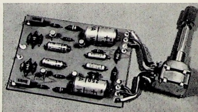
Bild 4. Ansicht des Basisbreitenreglers mit dem Potentiometer P1a, P1b
