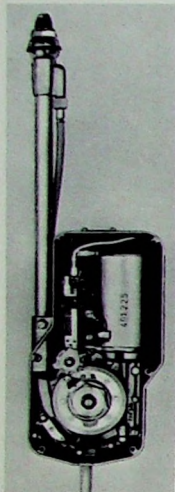
Antrieb der vollautomatischen Autoantenne „Auta 6000 H“ (Hirschmann)
