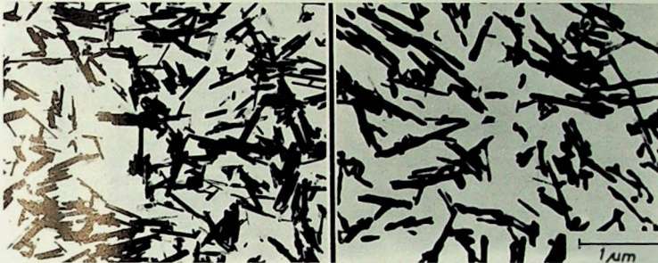
Bild 1. Größe und Schichtung der aktiven Partikel beim Chromdioxidband (links) und Eisenoxidband (rechts)
