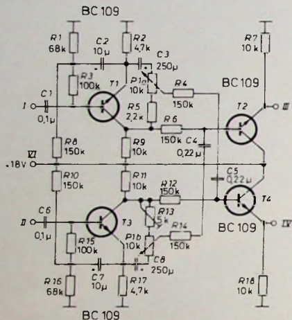
Bild 1. Schaltung des Basisbreitenreglers
