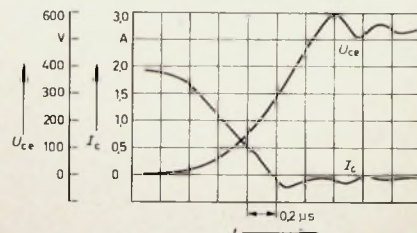
Bild 7. Abschaltverhalten des Schalttransistors BU 126 im Sperrwandlernetzteil
