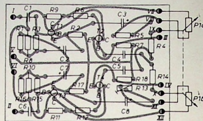
Bild 3. Anordnung der Bauteile auf der Platine
