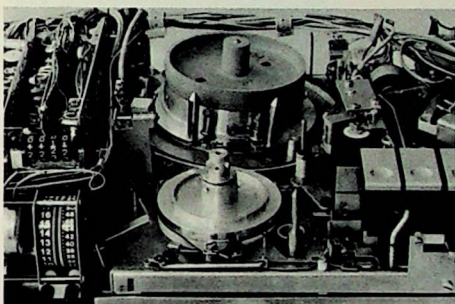
Bild 1 (oben). Video-Cassetten-Recorder „Optacord 700 Color VCR“ (Loewe-Opta)
