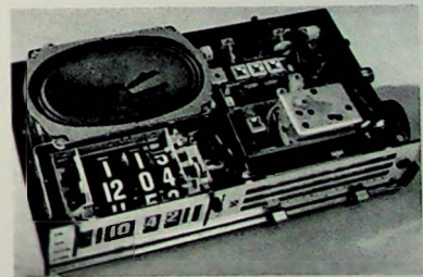
Innenansicht des „sono-clock 20“ (Grundig)
